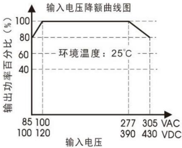
图 2 ) AC 输入电压降额_ 输出负载降额对应输入电压
